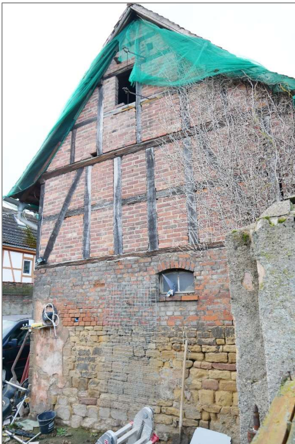
Nebengebäude 2 - Nordansicht
