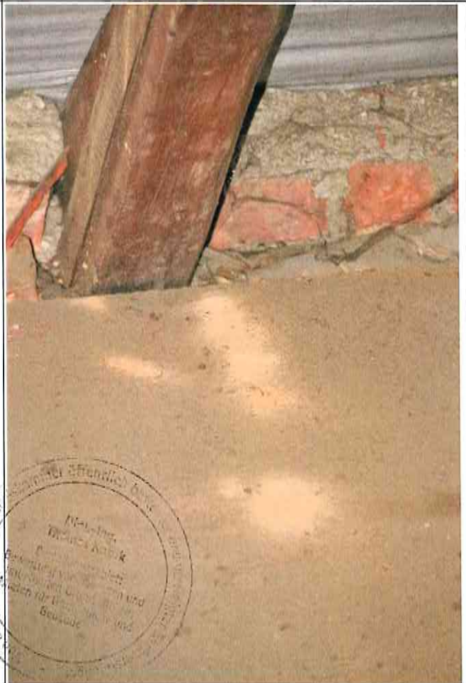
Dachgeschoss- Befall durch tierische Holzschädlinge
