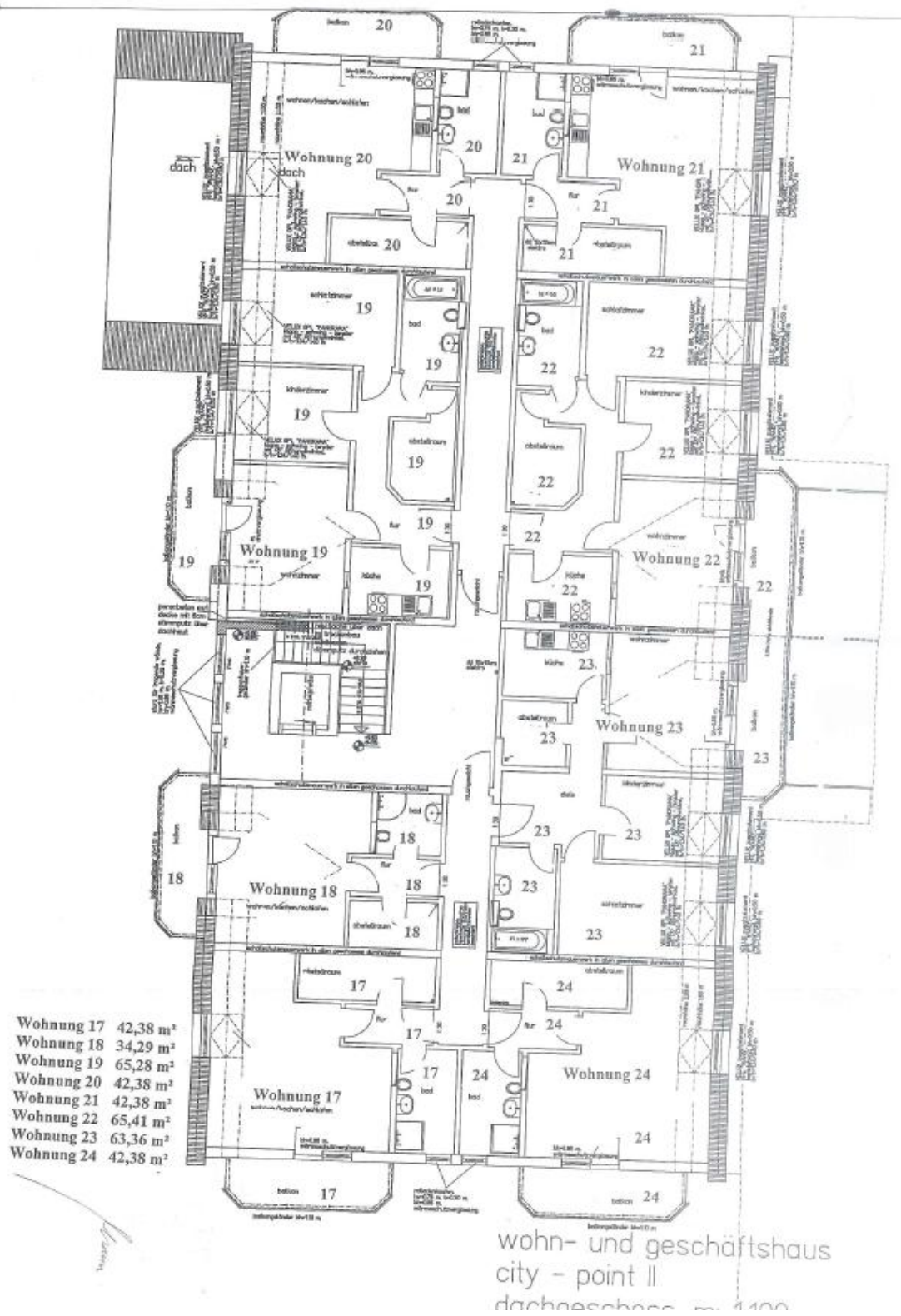
Grundriss Dachgeschoss
