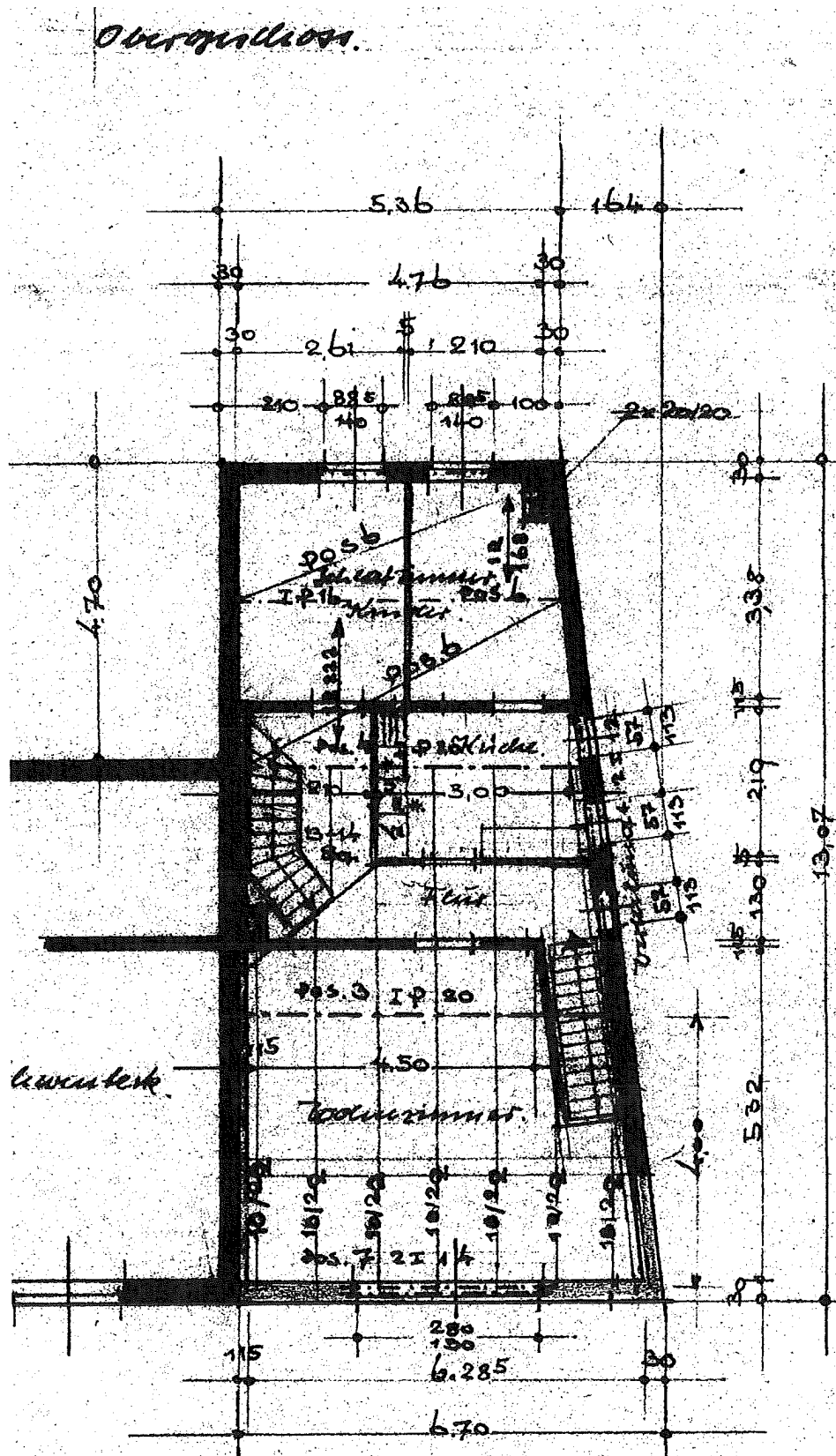
Grundriss OG
