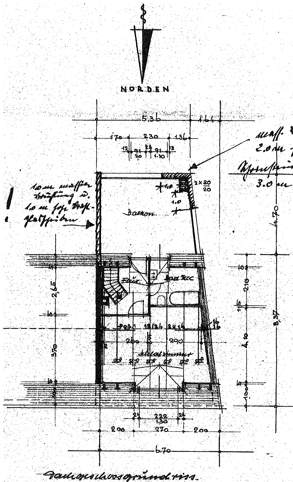
Grundriss DG
