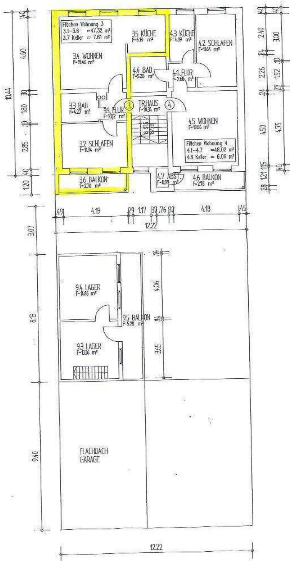
Grundriss 1. Obergeschoss (unmaßstäblich)
