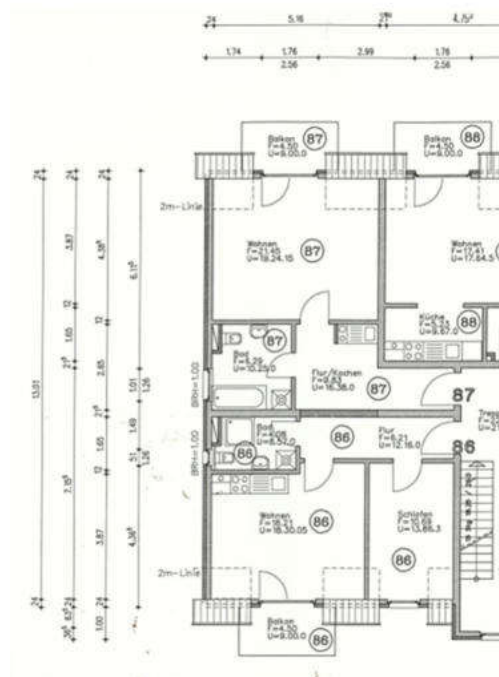
Grundriss Dachgeschoss mit Wohnungseigentum Nr. 87 gemäß Teilungserklärung und Aufteilungsplan
