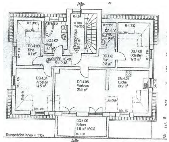
Foto 6: Grundriss WET Nr. 4
