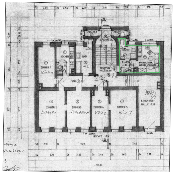
Grundriss Wohnung Nr. 2 gemäß ATP, ohne Maßstab
