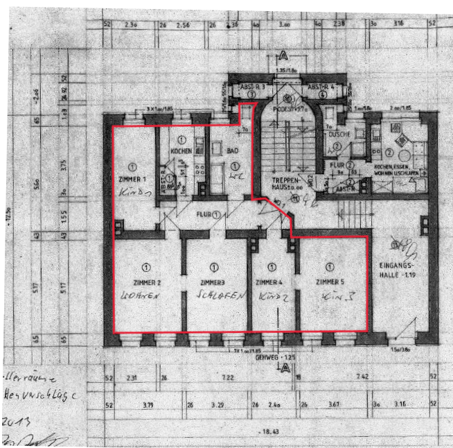
Grundriss Wohnung Nr. 1 gemäß ATP, ohne Maßstab
