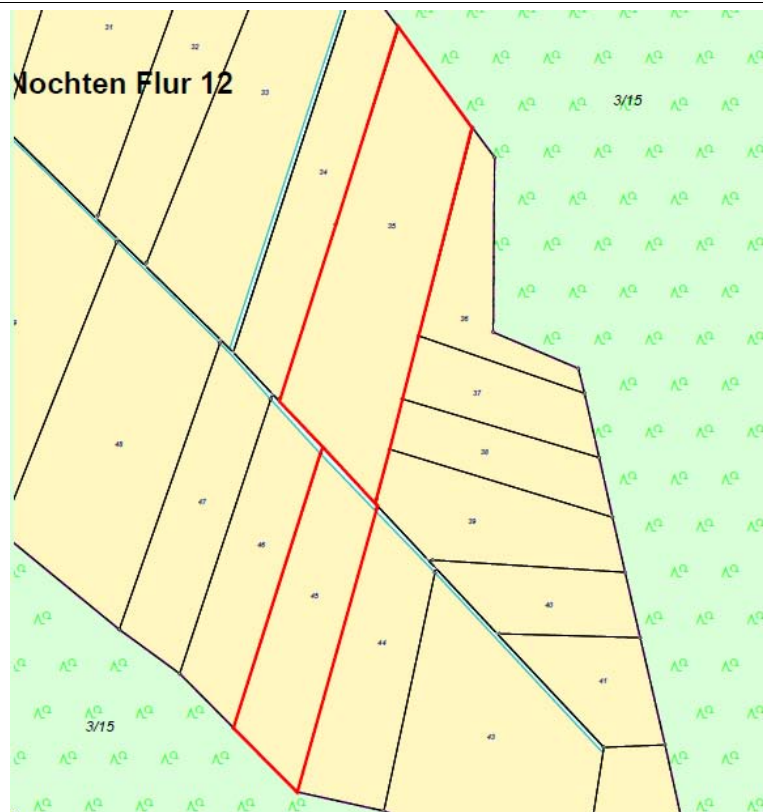
Ausschnitt aus der Flurkarte der Gemarkung Nochten mit Kennzeichnung der Flurstücke 35 und 45
