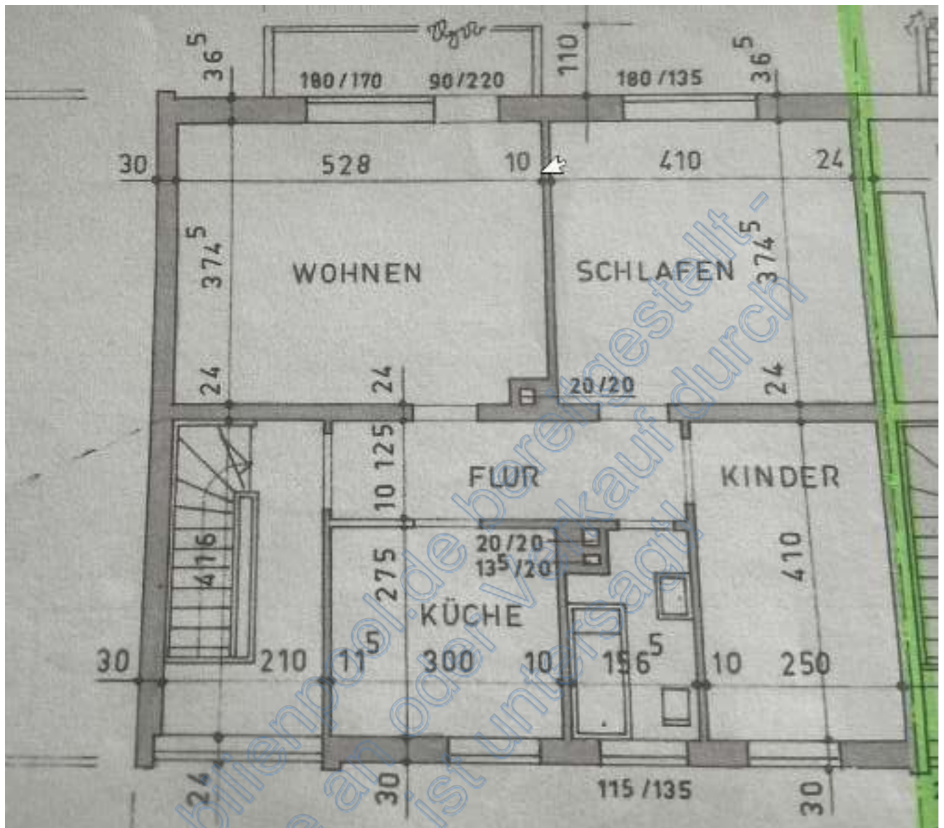
Grundriss Obergeschoss
