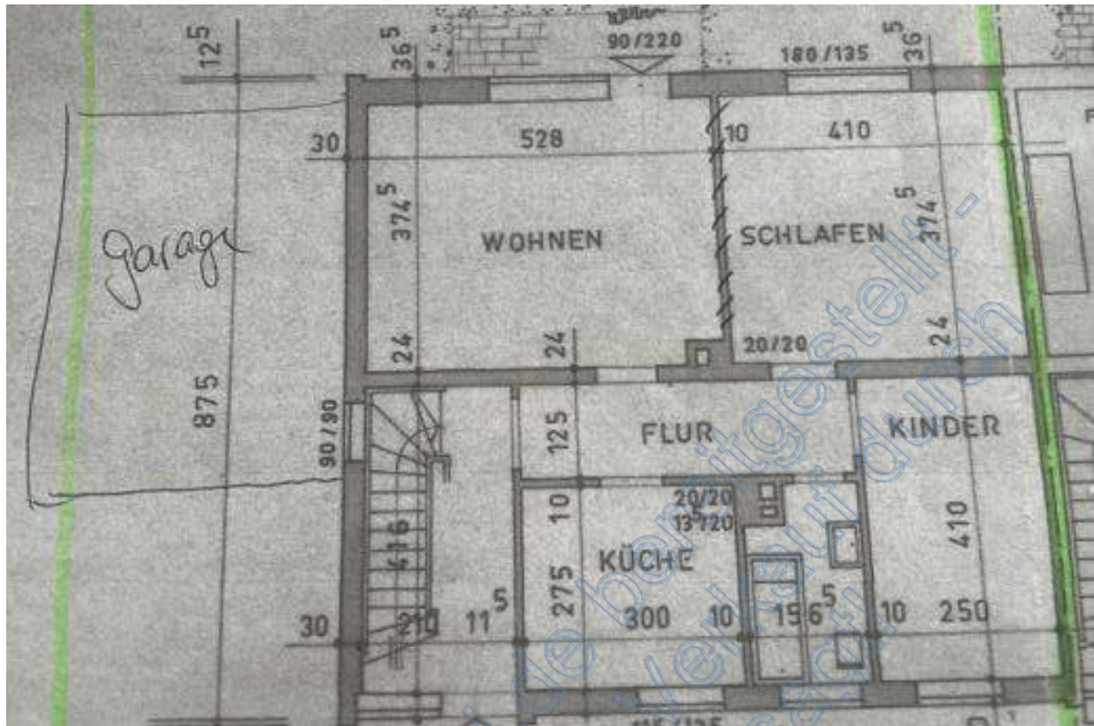
Grundriss EG
