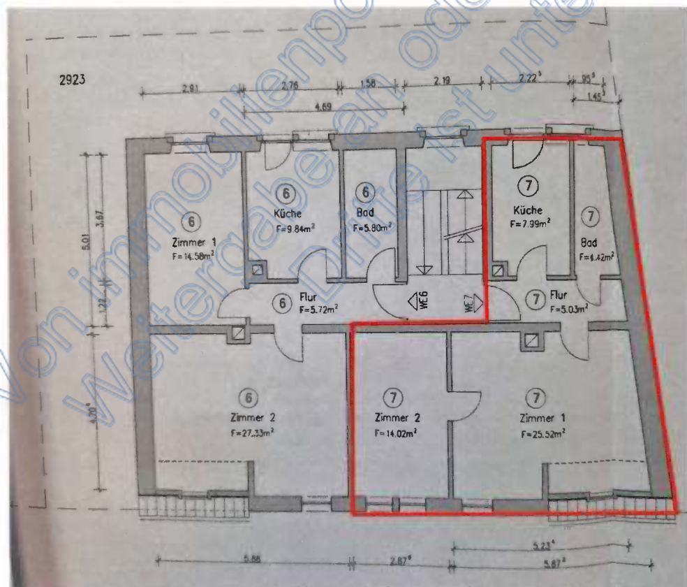
Grundriss Wohnung Nr. 7
