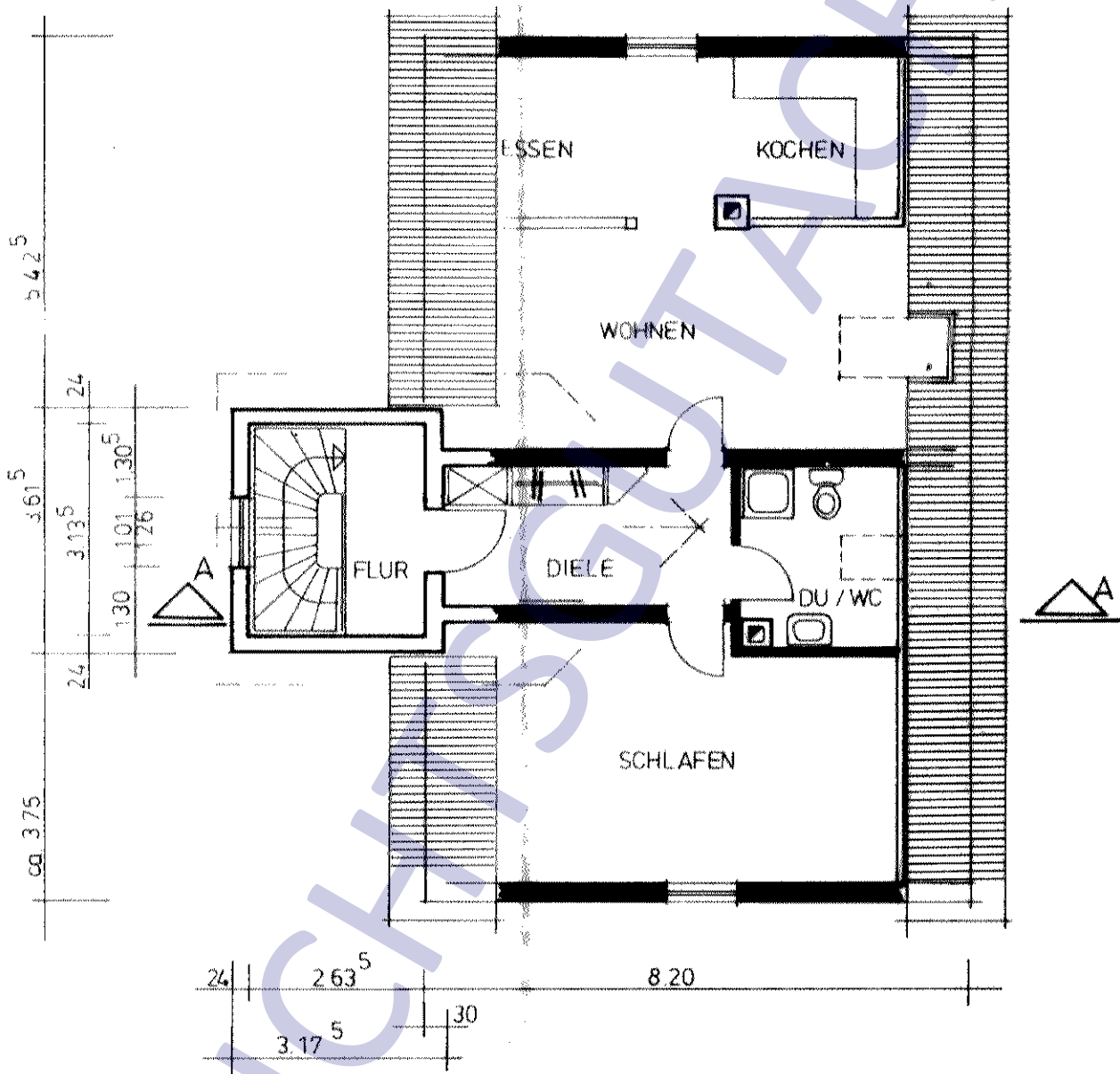
DACHGESCHOSS
