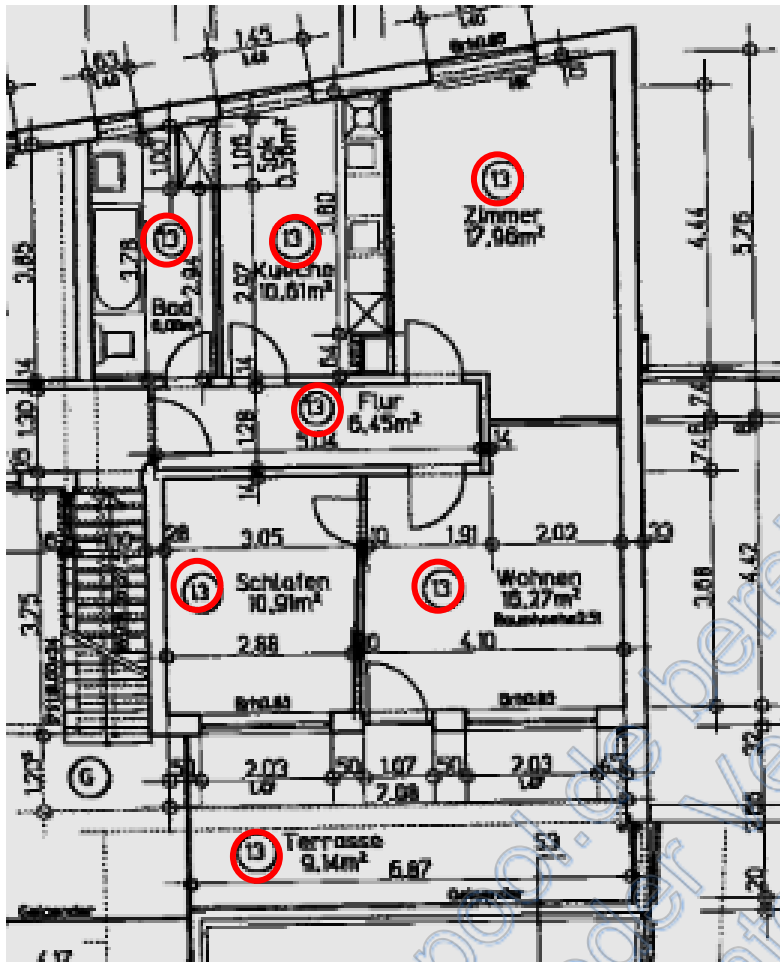
Grundriss WE 13 im DG
