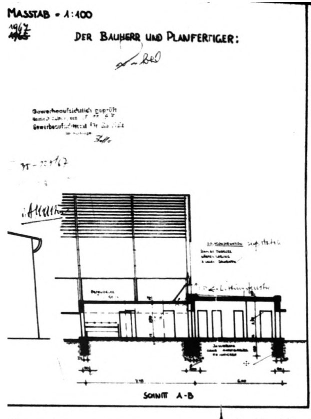
Anbau nach Norden gem. Genehmigungsunterlagen (oben) Schnitt (unten)
