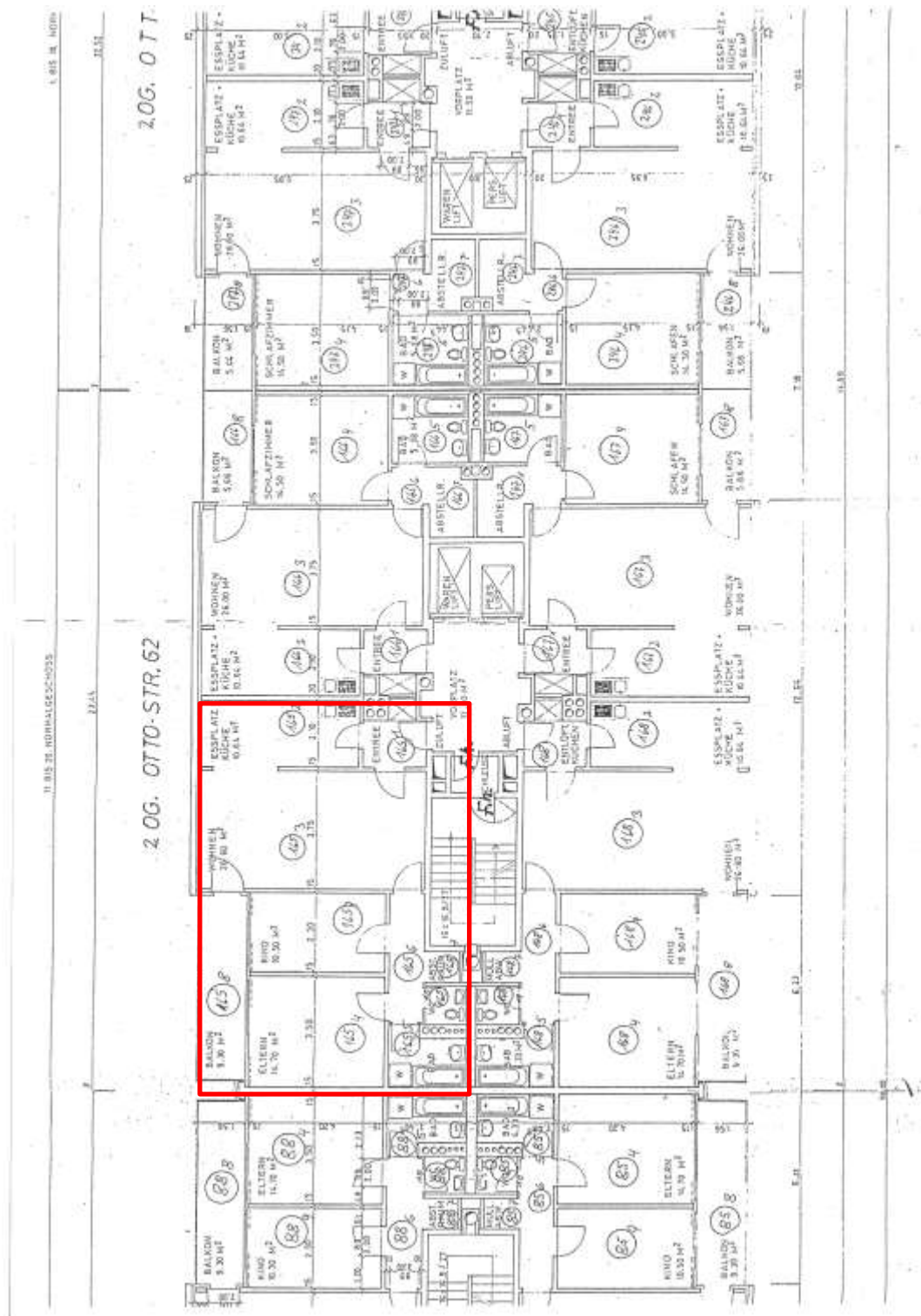
Grundriss 1: 2. Obergeschoss, SE-Nr. 165
