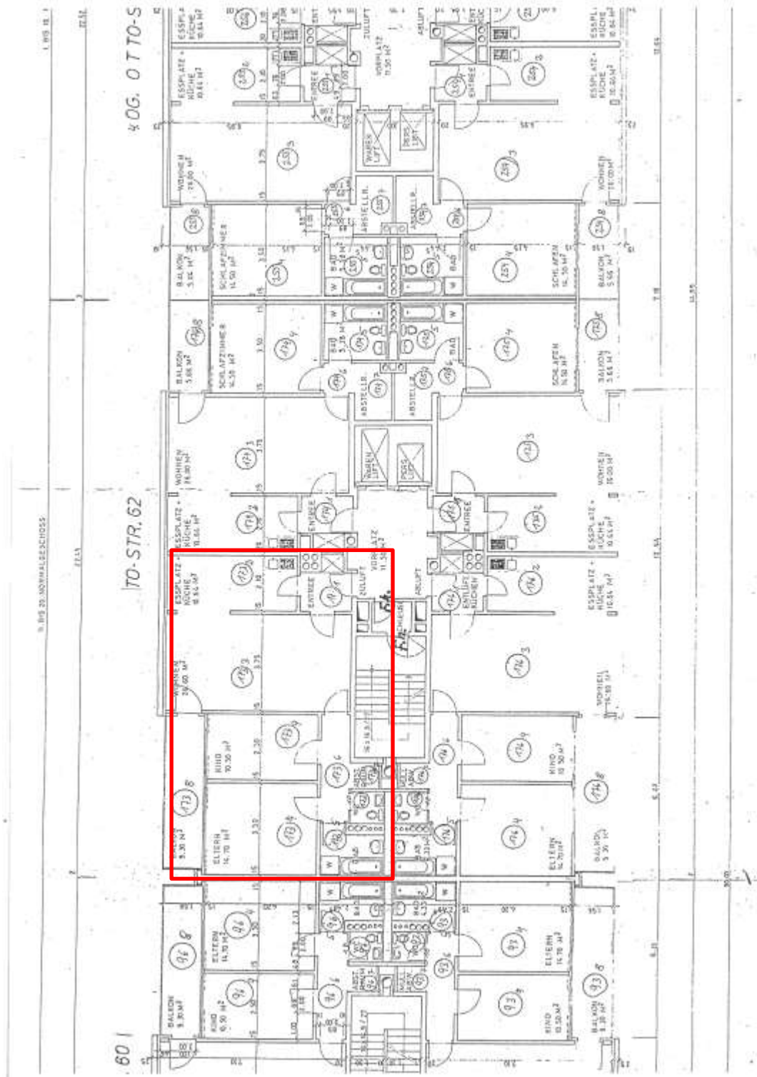
Grundriss 1: 4. Obergeschoss, SE-Nr. 173
