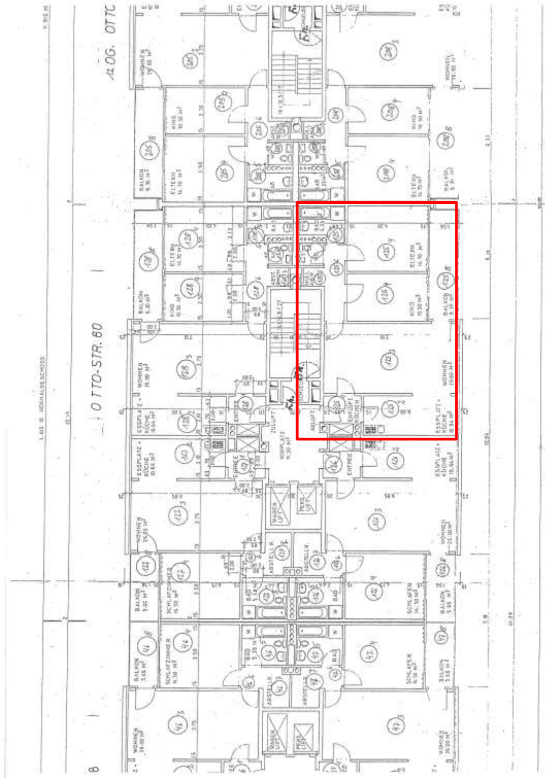
Grundriss 1: 12. Obergeschoss, SE-Nr. 125
