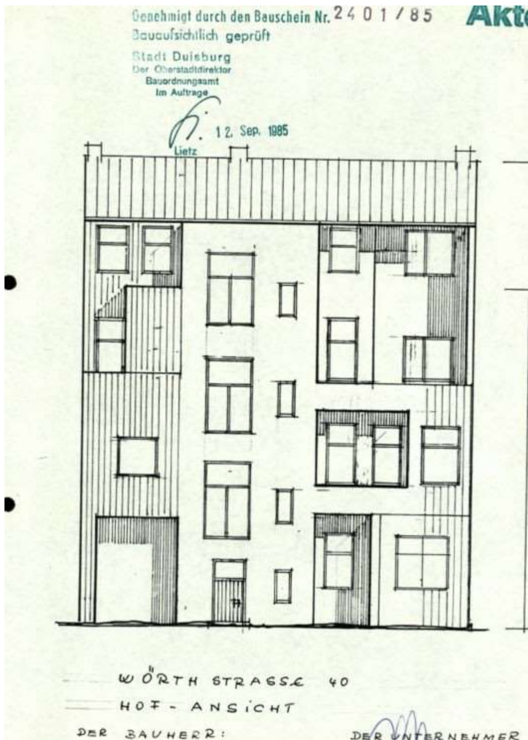
Bild 2: Rückansicht Quelle: Bauakte der Stadt Duisburg
