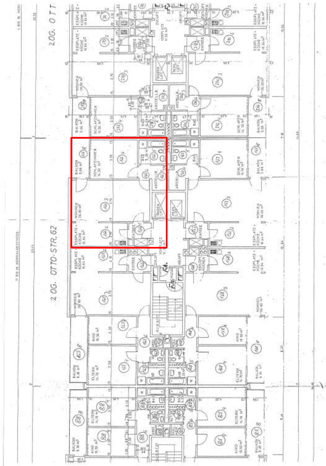
Grundriss 1: 2. Obergeschoss, SE-Nr. 166
