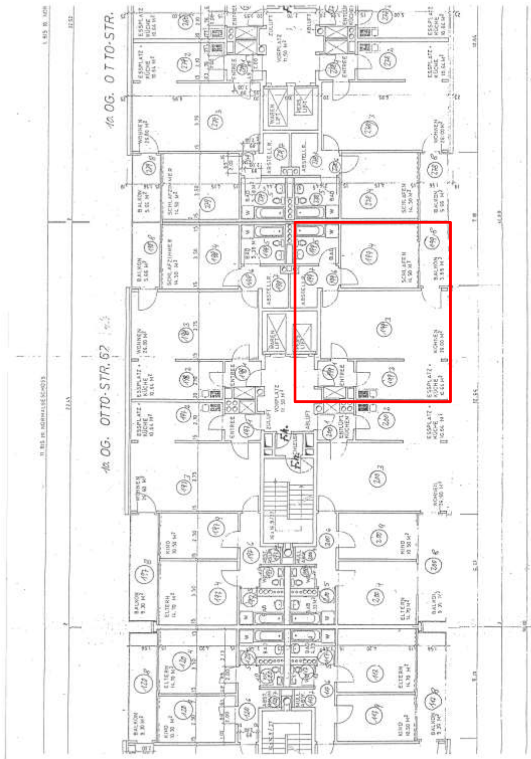
Grundriss 1: 10. Obergeschoss, SE-Nr. 199
