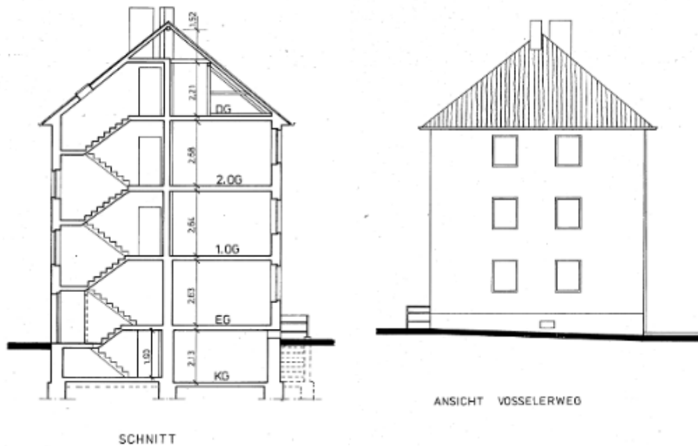
Schnitte / Ansichten
