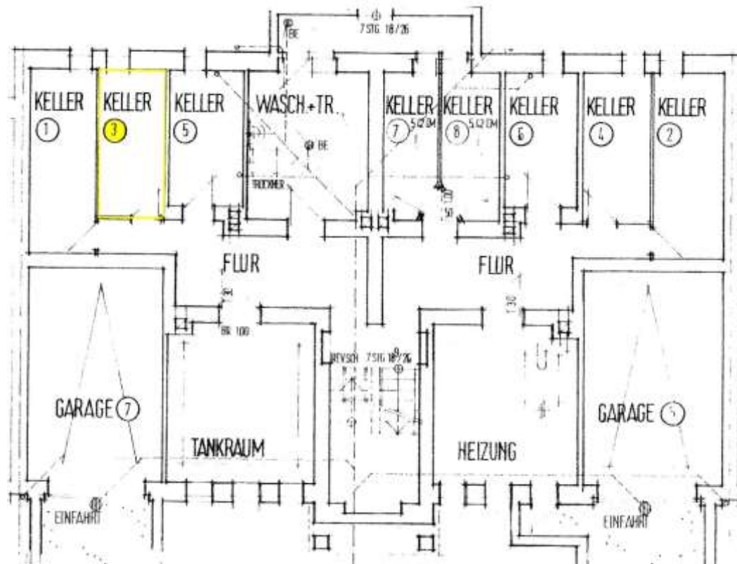
Grundriss Kellergeschoss mit dem zum Wohnungseigentum Nr. 3 gehörenden Keller- raum gemäß Teilungserklärung
