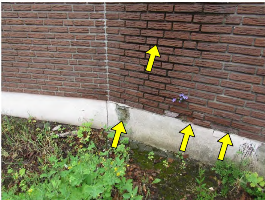
Foto 10: Zufahrt, Trennwand mit beschädigten Fugen und Abplatzungen an den Ziegelsteinen und dem Putz
