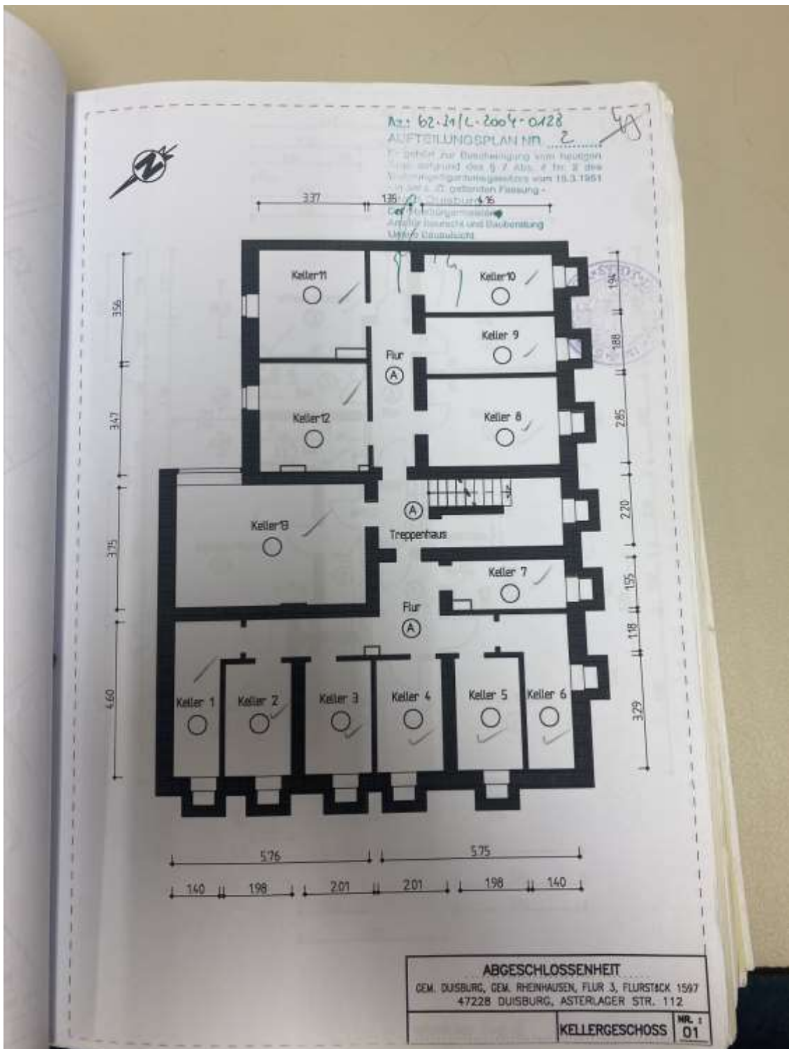
Bild 1: Kellergeschoss Quelle: Teilungserklärung Grundakte AG Duisburg
