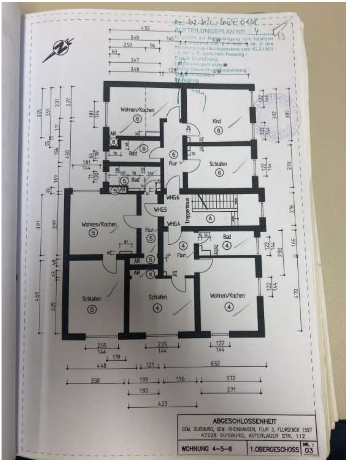
Bild 2: 1. OG SE Nr. 5 Quelle: Teilungserklärung Grundakte AG Duisburg
