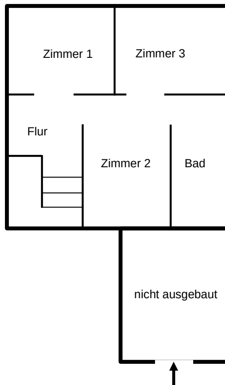
Zeichnung 3: Grundriss Dachgeschoss
