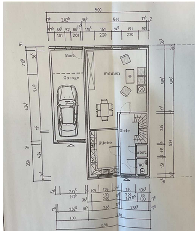
Zeichnung 1: Grundriss Erdgeschoss
