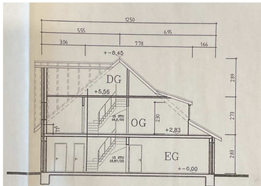
Zeichnung 4: Gebäudeschnitt
