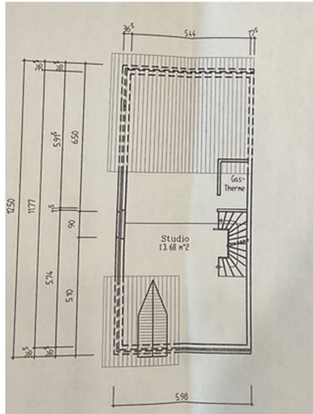
Zeichnung 3: Grundriss Spitzboden
