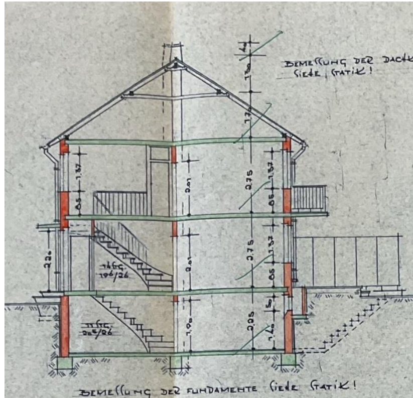
Zeichnung 4: Gebäudeschnitt
