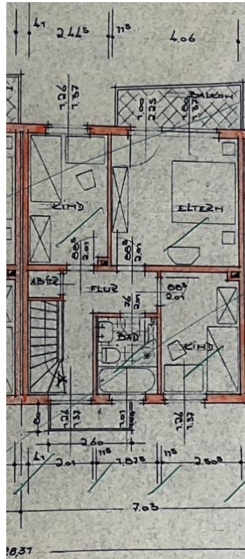
Zeichnung 3: Grundriss Obergeschoss
