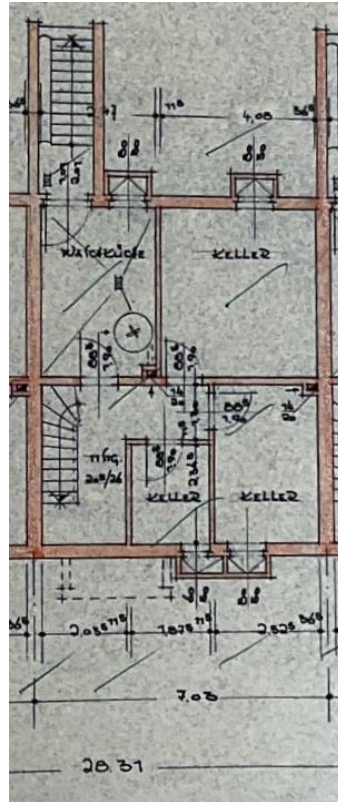
Zeichnung 1: Grundriss Kellergeschoss
