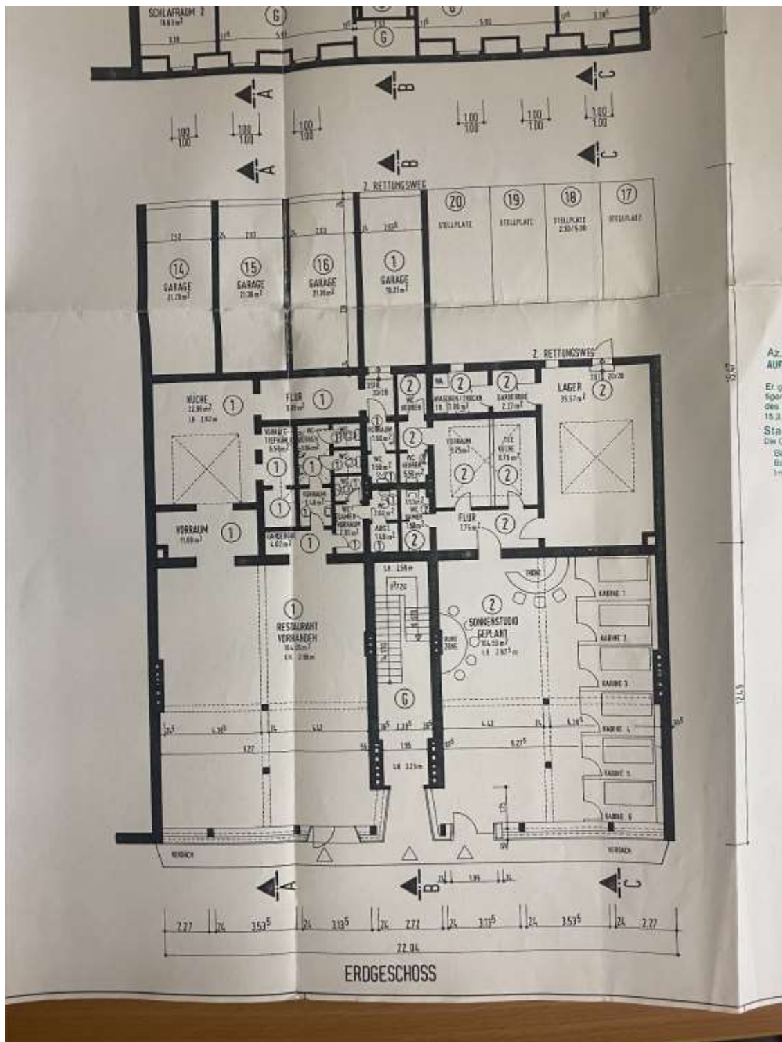
Bild 1: SE Nr. 1 im EG / Quelle: Aufteilungsplan Grundakte
