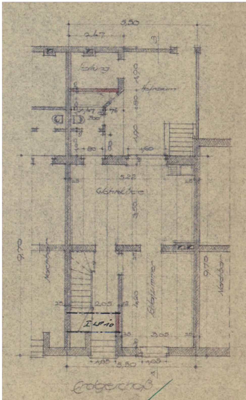
Grundriss Erdgeschoss gemäß Hausakte der Bauverwaltung
