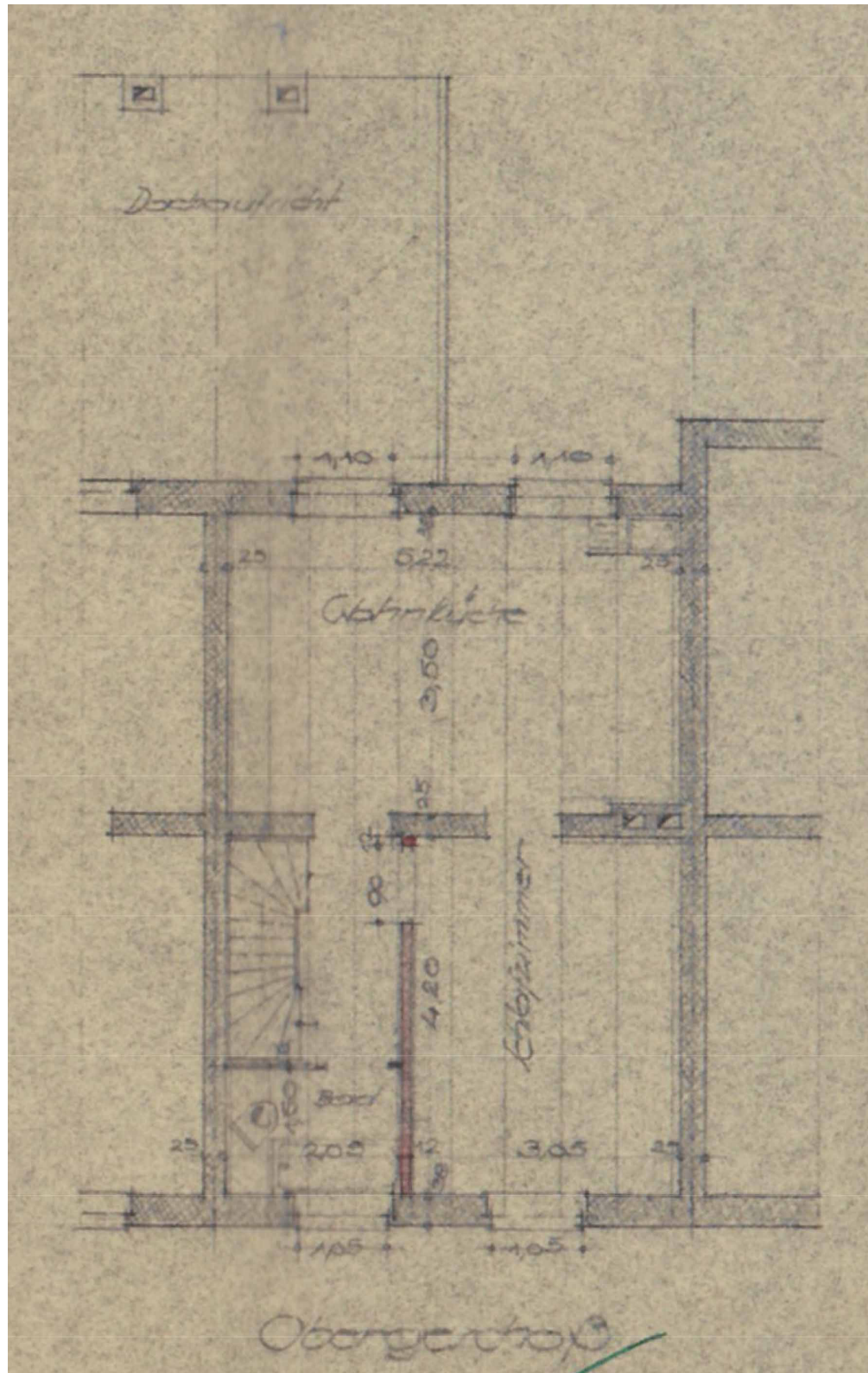
Grundriss Obergeschoss gemäß Hausakte der Bauverwaltung
