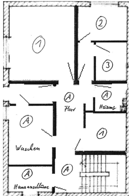
Kellergeschoss
