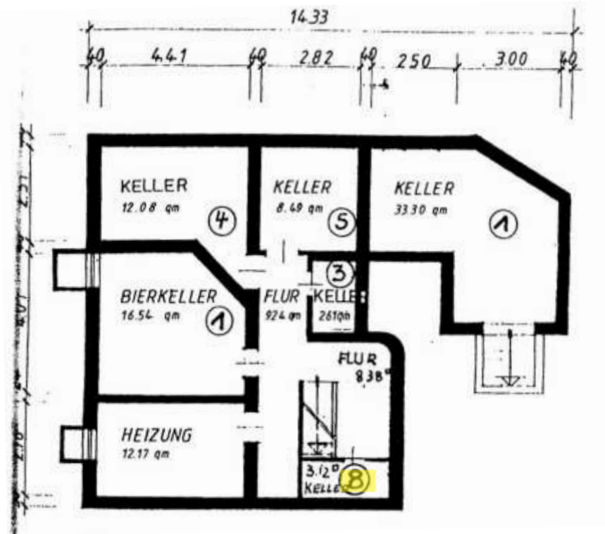
Grundriss Kellergeschoss
