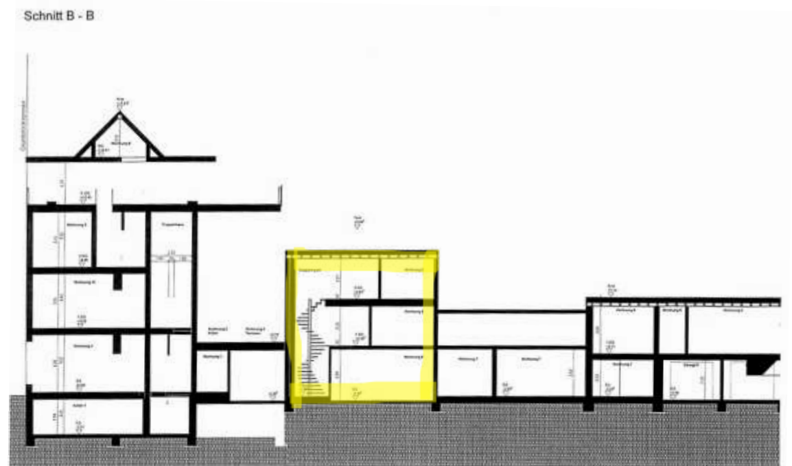
Vorderhaus Schnitt
