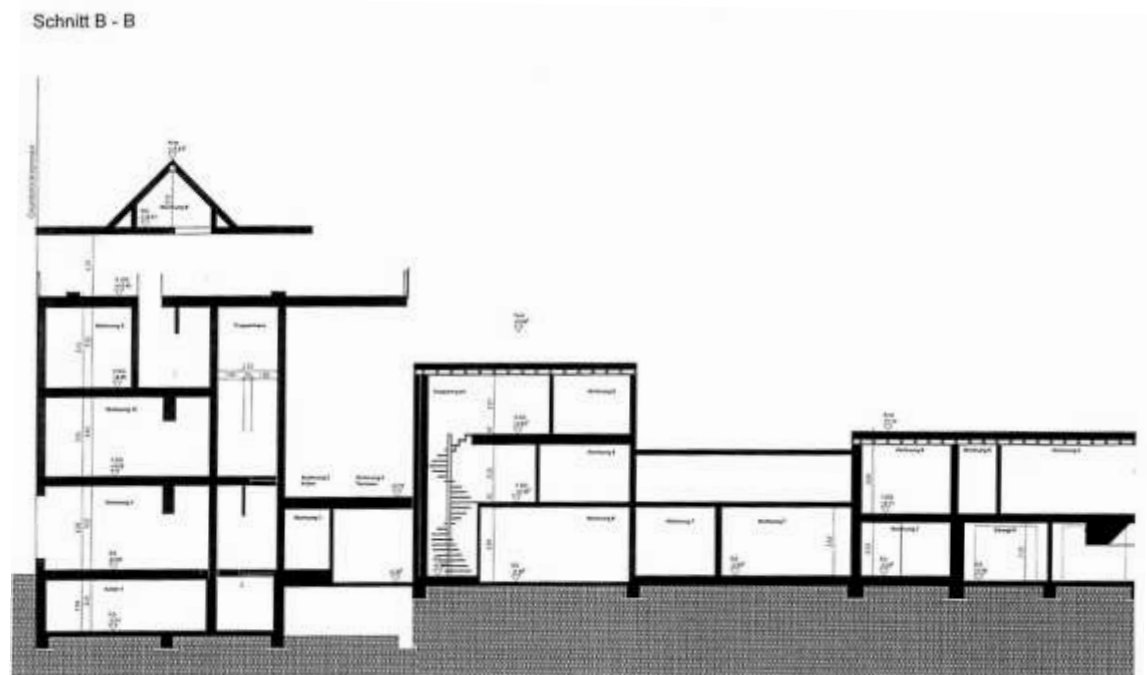
Vorderhaus Schnitt
