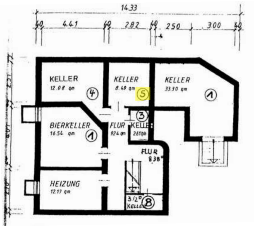
Grundriss Kellergeschoss
