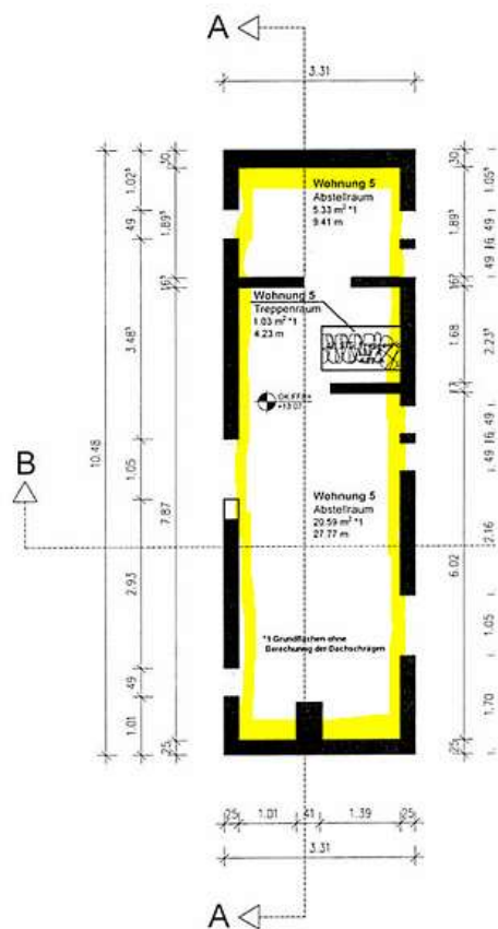
Grundriss Spitzboden- WE Nr. 5 – aus den Planunterlagen
