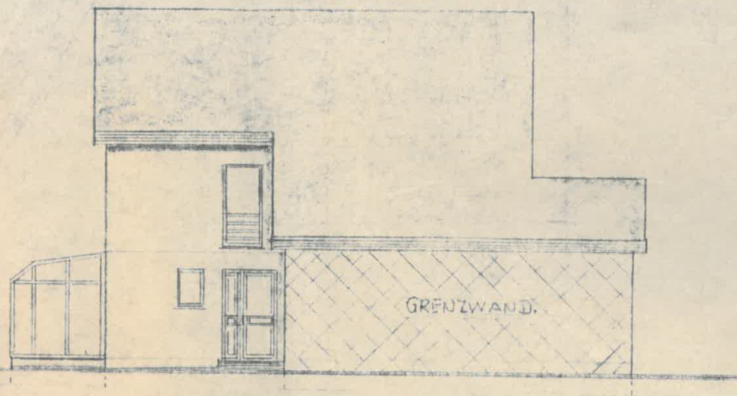
N.O.-ANSICHT:
