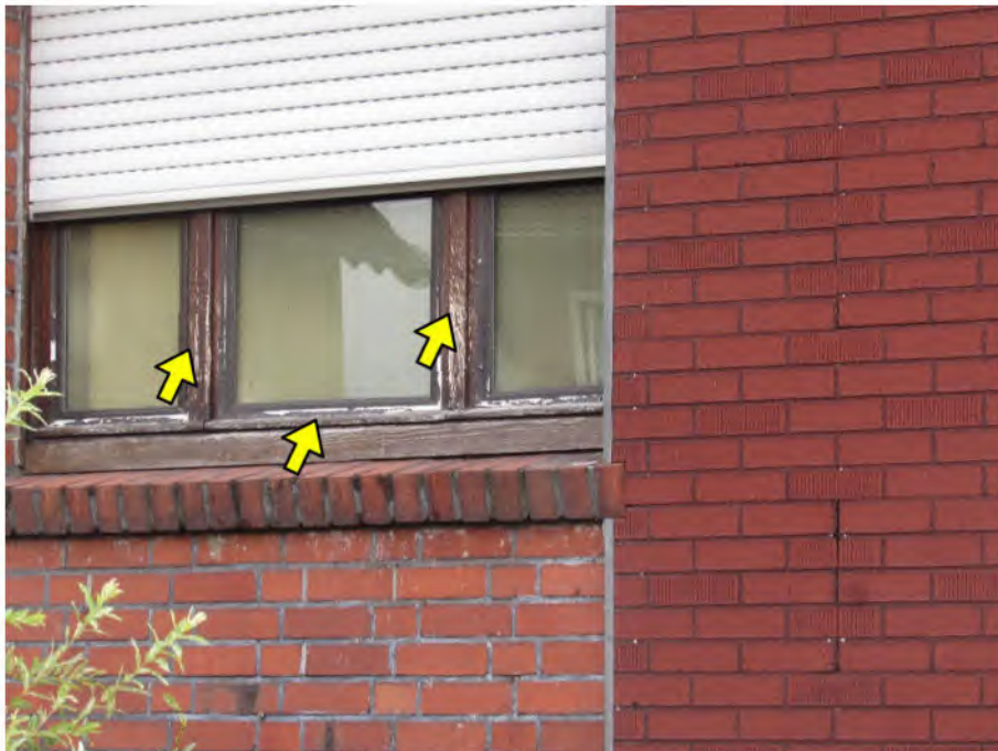
Foto 6: überalterte verwitterte Holzfenster
