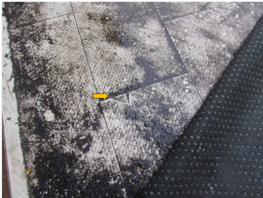
Foto 14: Terrasse, beschädigte Fliesen
