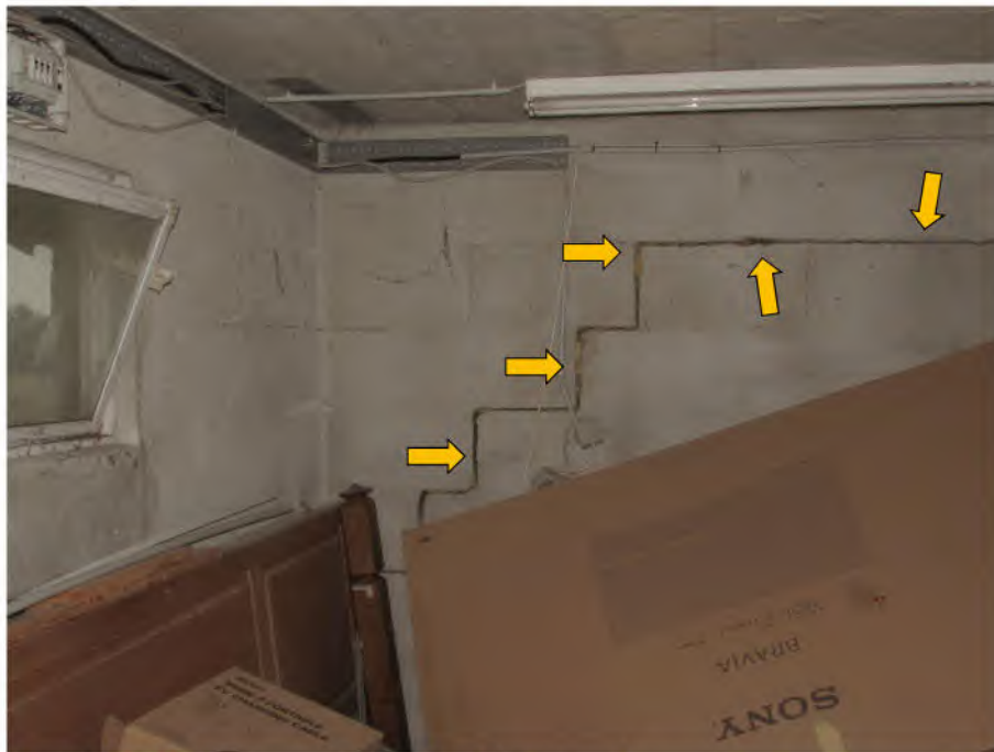
Foto 11: PKW-Garage, Risse im Mauerwerk
