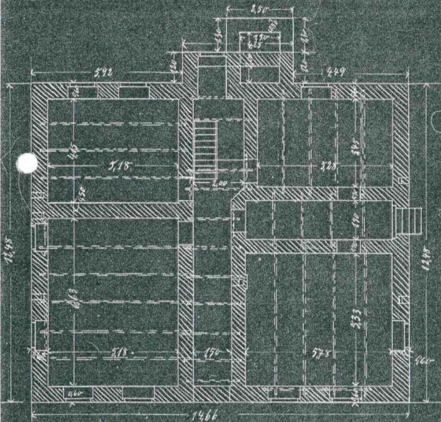
Hellengeschoss
