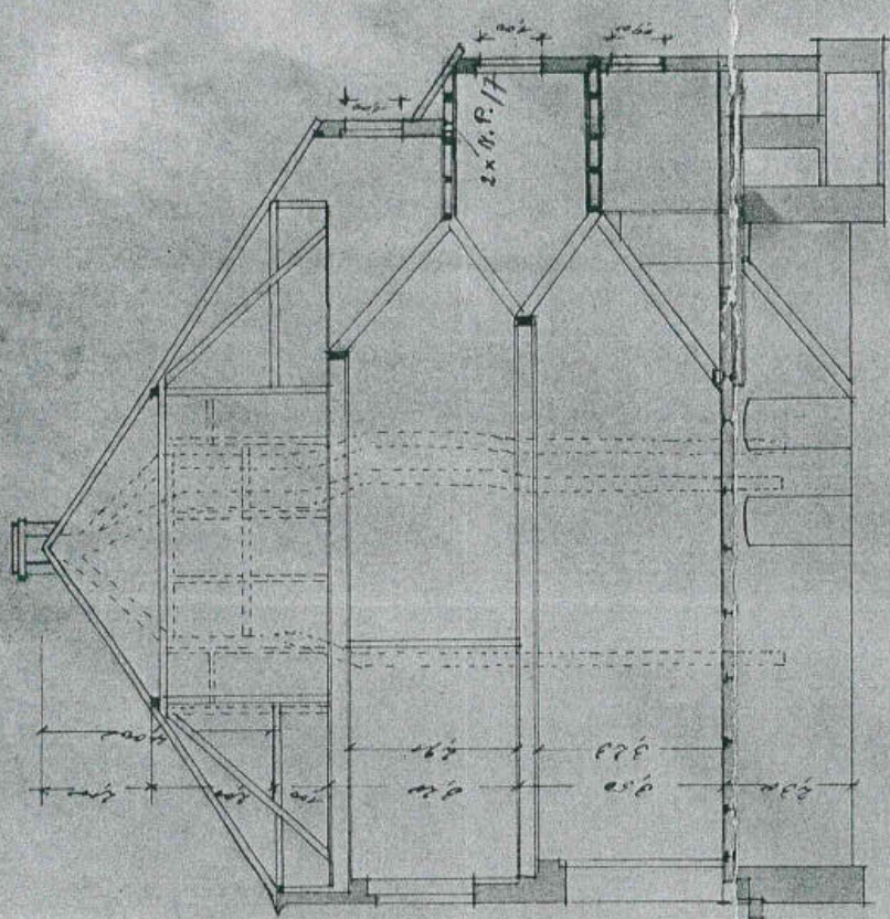
QUERSCHNITT
