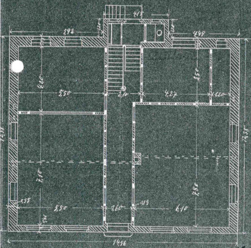
Erdgeschoss
