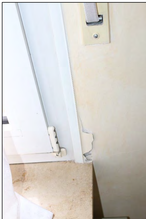
Foto Nr. 32: Erdgeschoss, WE Nr. 1, Esszimmer, Putzschaden
