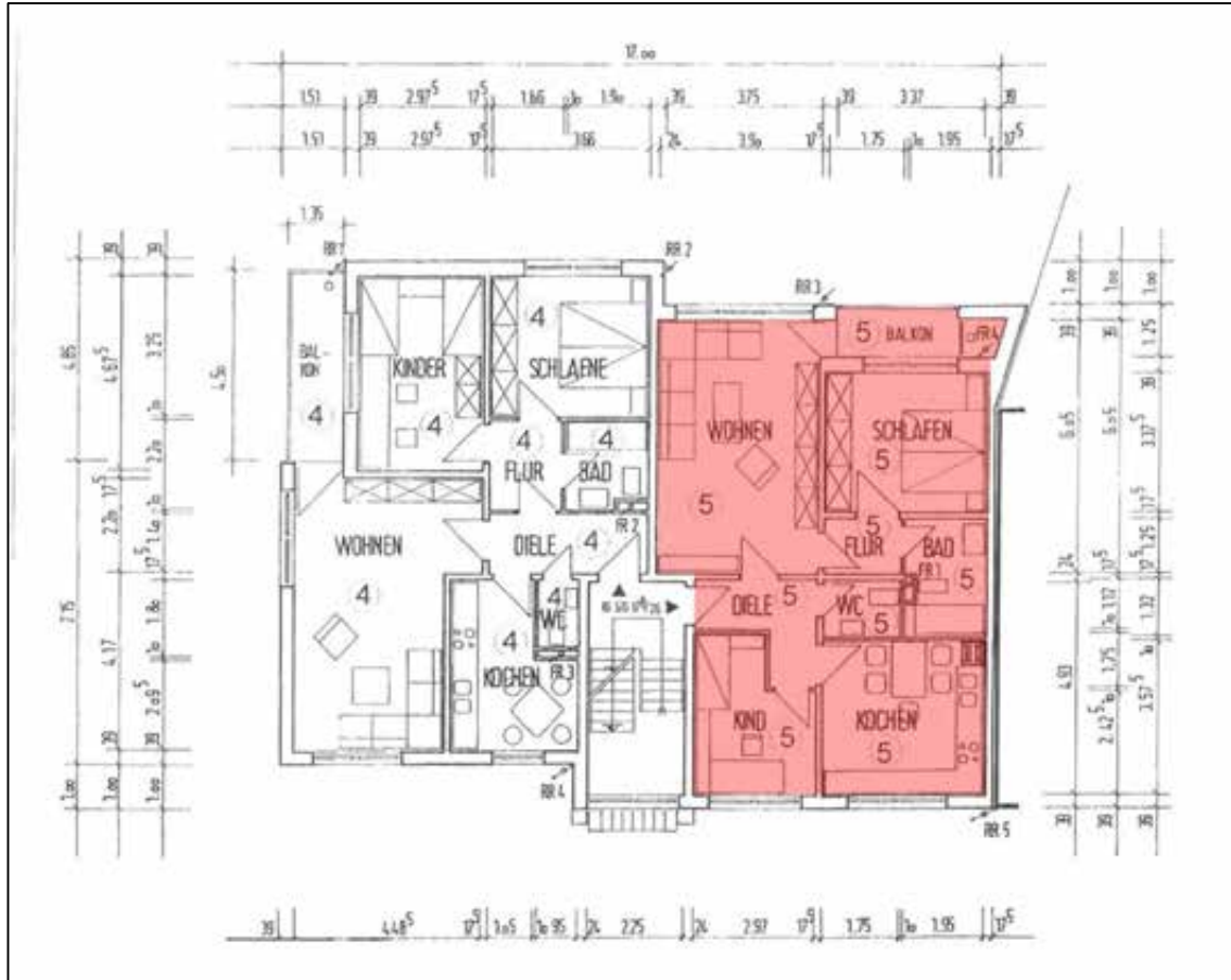
Abbildung 53 Grundriss vom 1. Obergeschoss Das zu bewertende Sondereigentum ist rot unterlegt, aus den Bauakten der Stadt Hamm, ohne Maßstab © Stadt Hamm
