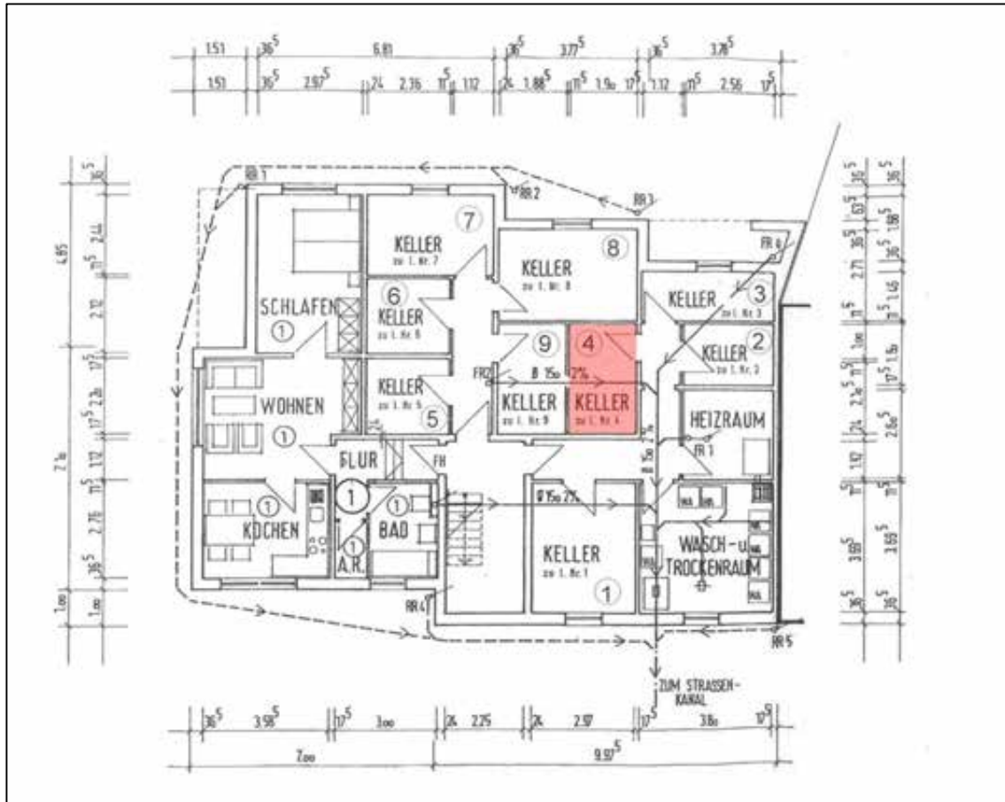
Abbildung 52 Grundriss vom Kellergeschoss Das zu bewertende Sondereigentum ist rot unterlegt, in der Örtlichkeit modifiziert, stimmt mit den Angaben der Teilungserklärung nicht überein aus den Bauakten der Stadt Hamm, ohne Maßstab © Stadt Hamm
