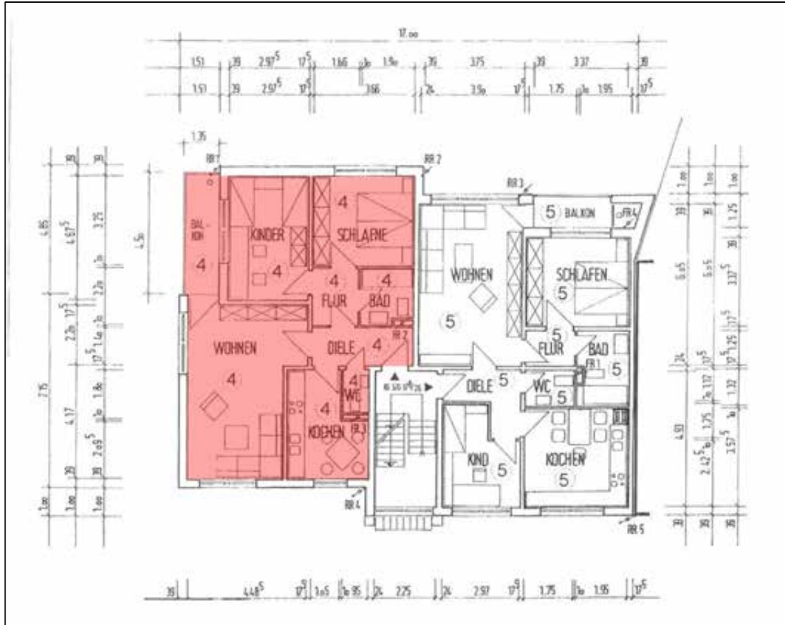
Abbildung 51 Grundriss vom 1. Obergeschoss Das zu bewertende Sondereigentum ist rot unterlegt, aus den Bauakten der Stadt Hamm, ohne Maßstab © Stadt Hamm
