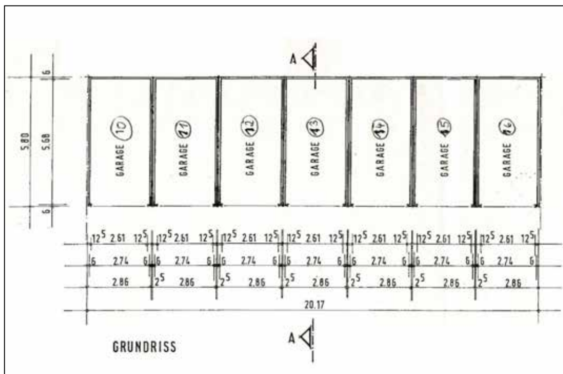
Abbildung 43 Grundriss vom Garagengebäude aus den Bauakten der Stadt Hamm, ohne Maßstab © Stadt Hamm
