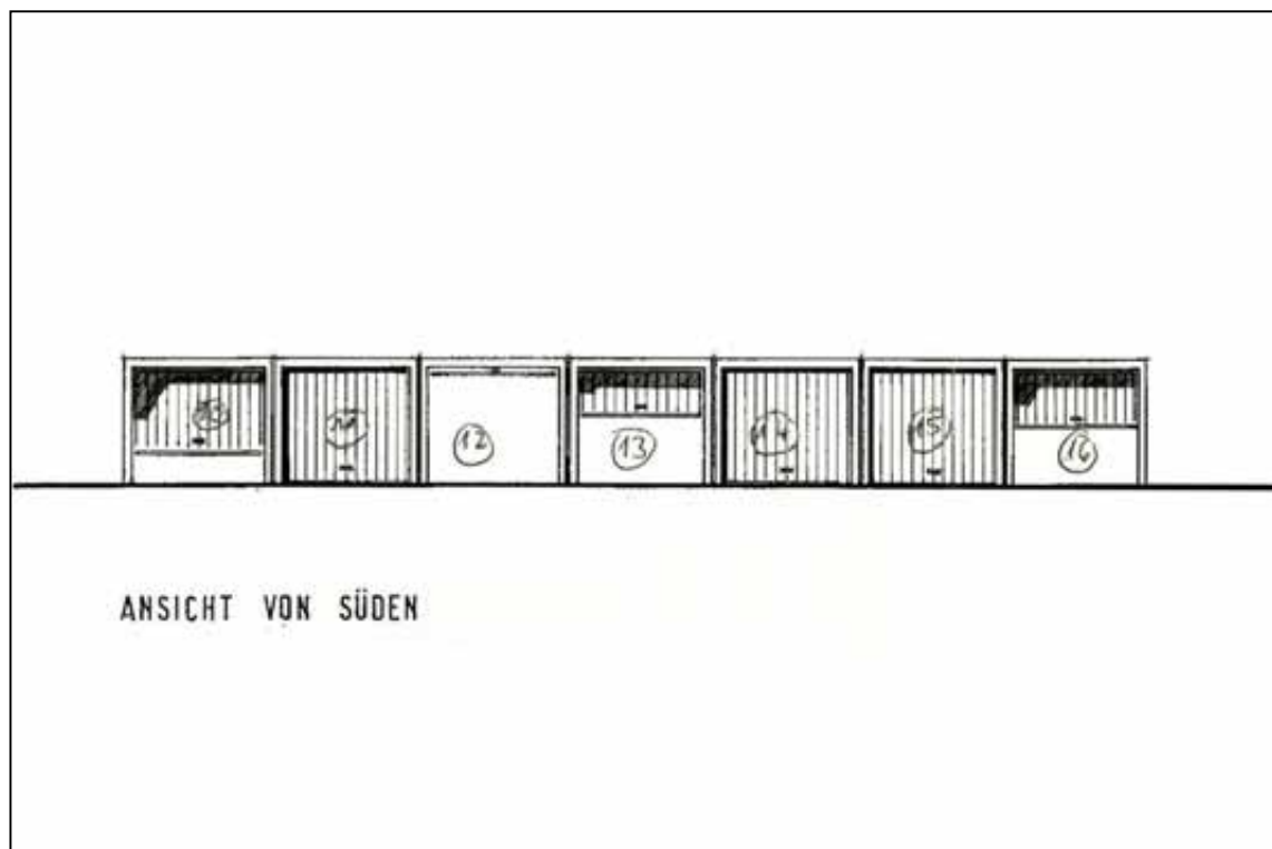
Abbildung 41 Ansicht vom Garagengebäude aus den Bauakten der Stadt Hamm, ohne Maßstab © Stadt Hamm
