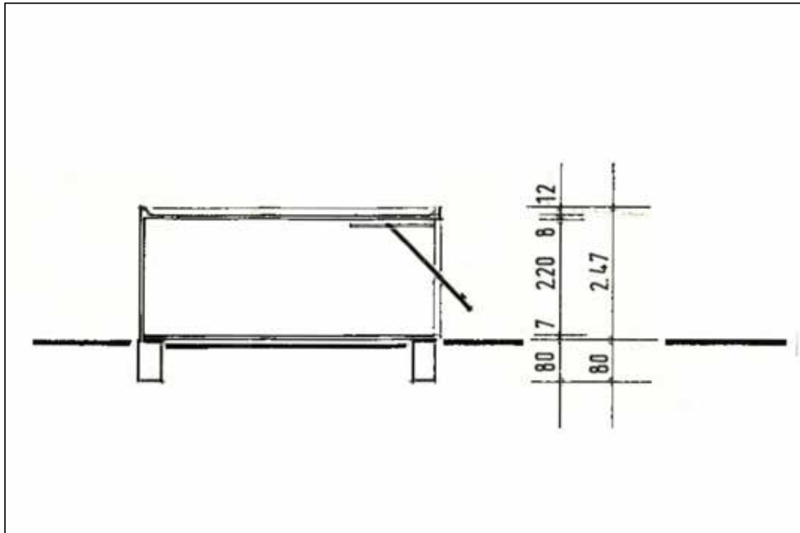
Abbildung 42 Schnitt durch das Garagengebäude aus den Bauakten der Stadt Hamm, ohne Maßstab © Stadt Hamm
