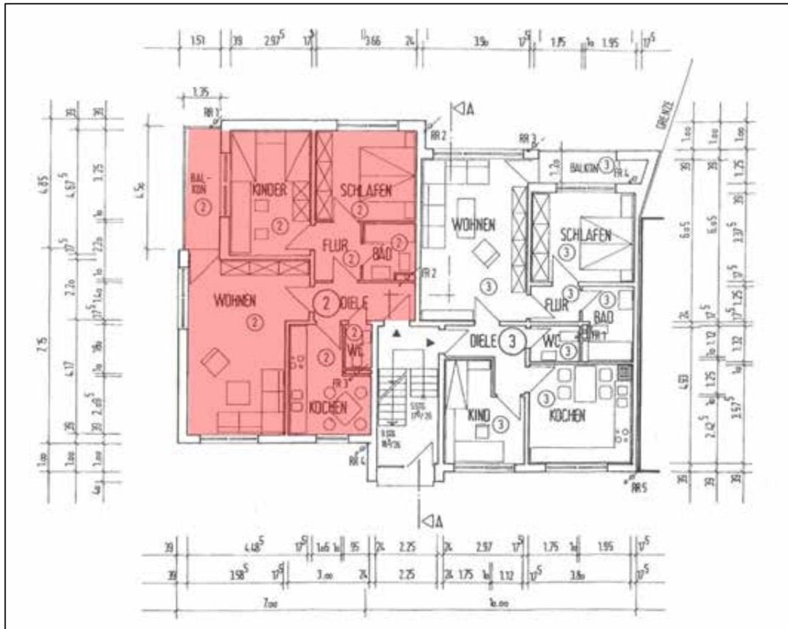
Abbildung 53 Grundriss vom Erdgeschoss Das zu bewertende Sondereigentum ist rot unterlegt, aus den Bauakten der Stadt Hamm, ohne Maßstab © Stadt Hamm
