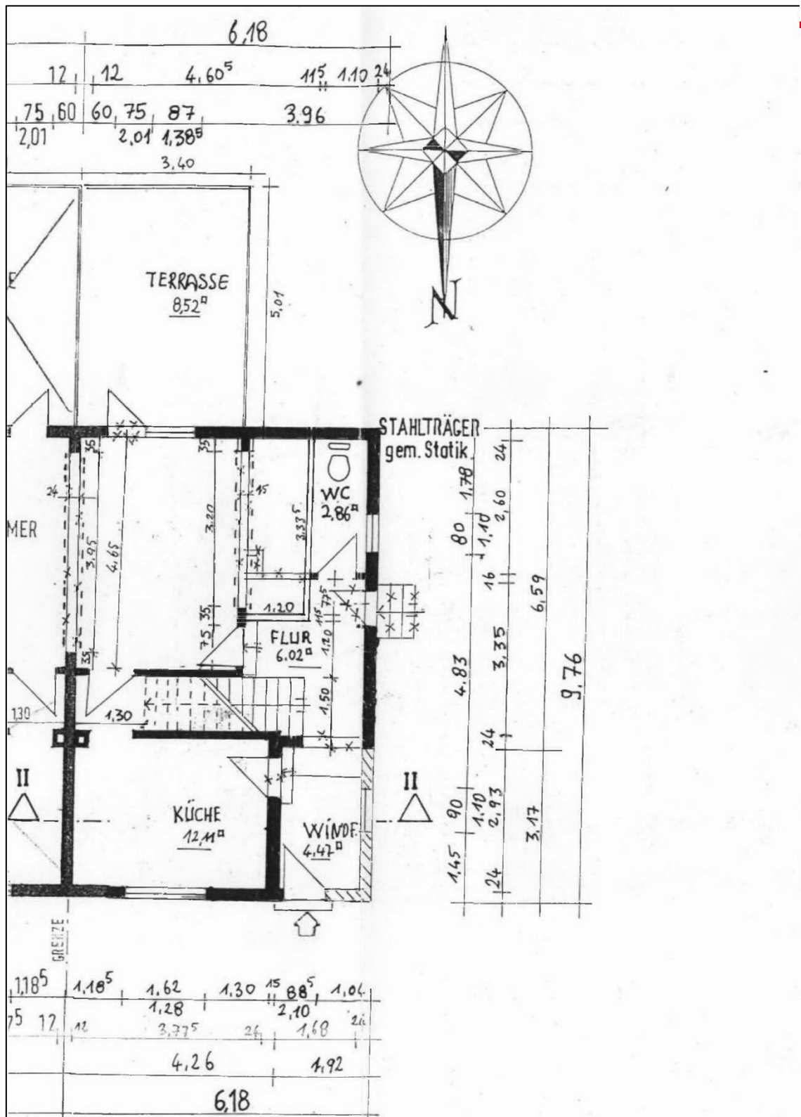
Abbildung 13 Erdgeschossgrundriss der Einfamilien-Doppelhaushälfte ohne Maßstab, in der Örtlichkeit modifiziert. aus den Bauakten der Stadt Hamm © Stadt Hamm
