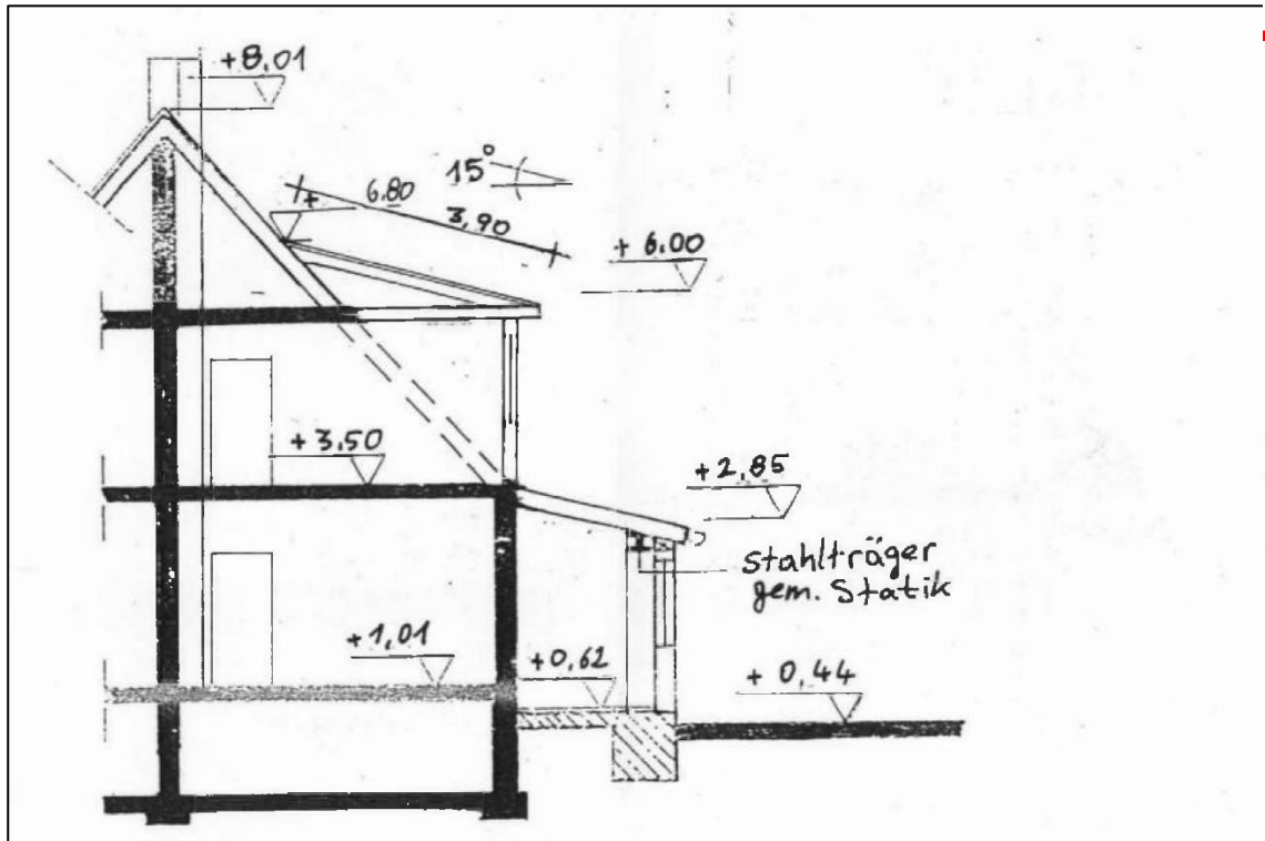
Abbildung 15 Schnitt durch die Einfamilien-Doppelhaushälfte Maßstab 1 : 100 aus den Bauakten der Stadt Hamm © Stadt Hamm
