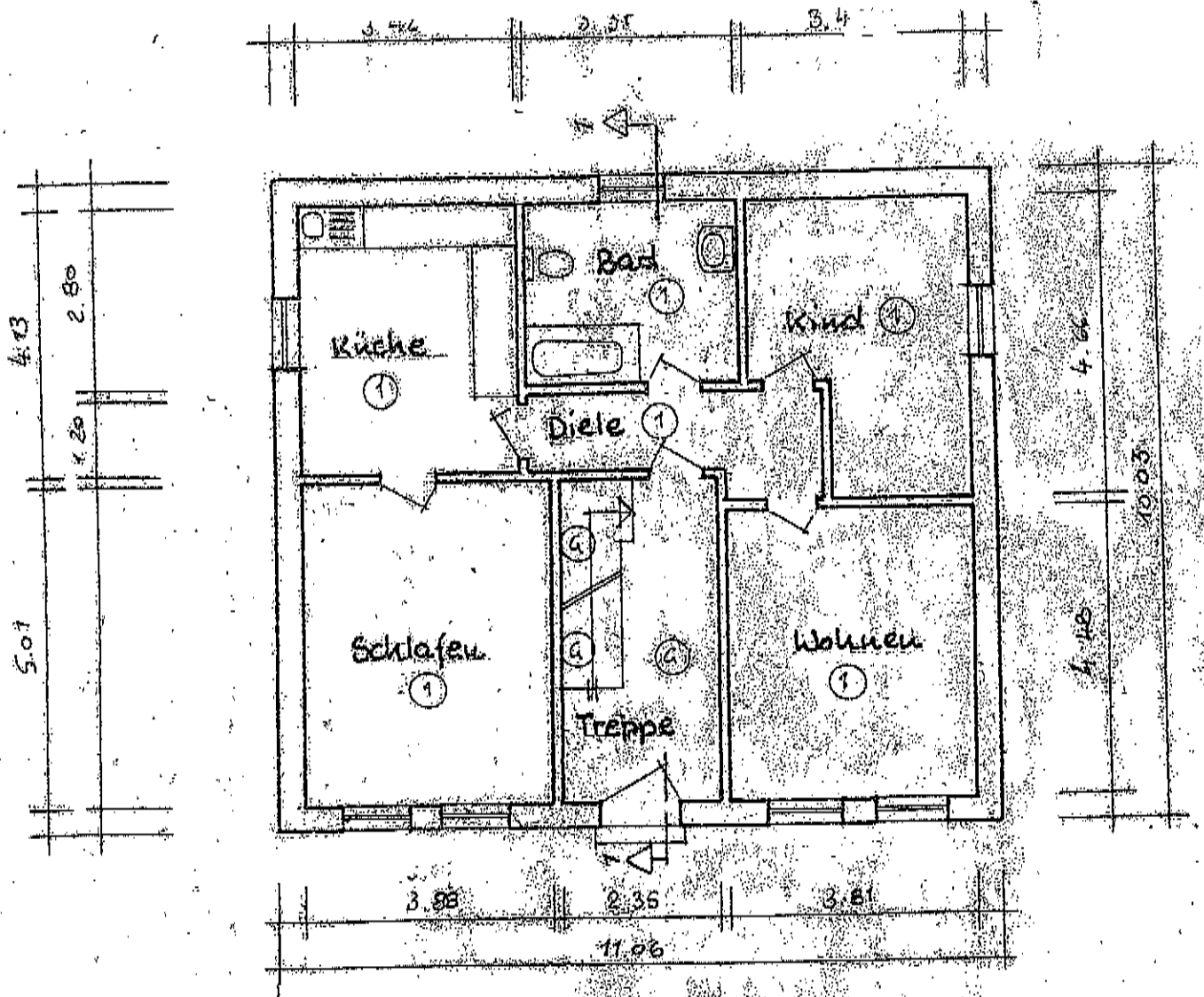
ERDGESCHOSS
