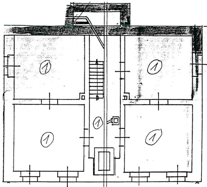
Kellergeschoss
