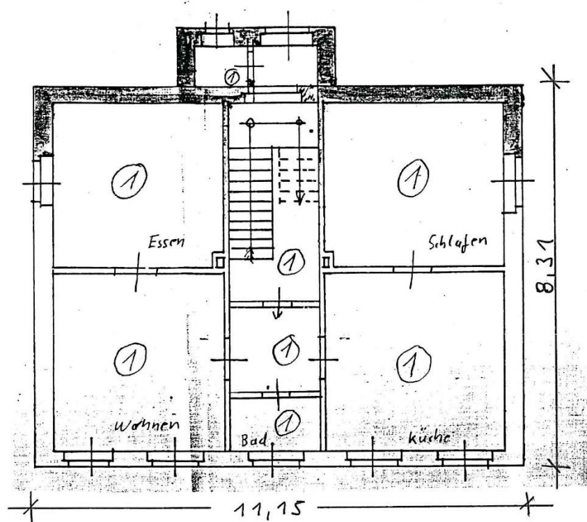
1. Obergeschoss
