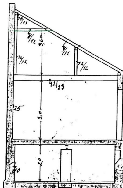
Schnitt Anbau
