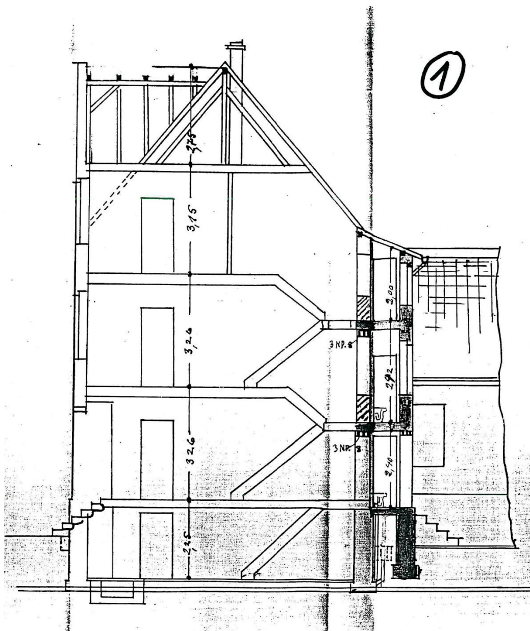
Schnitt
