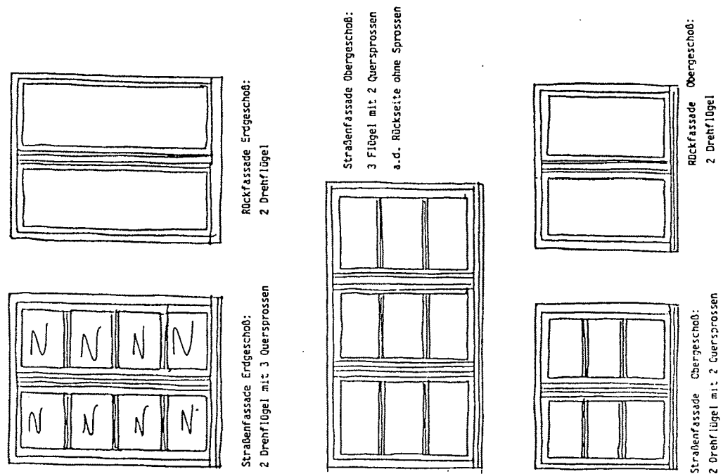
Anlage 2.3 Fenster für Haustypen IV und V
