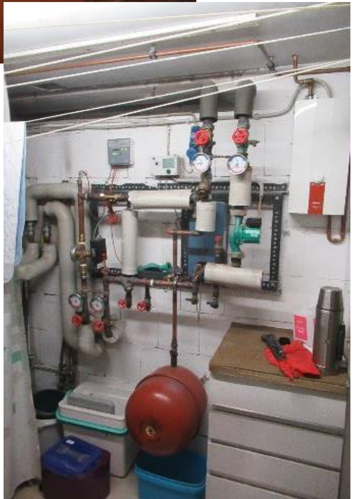
Fernwärmeüber- gabestation
