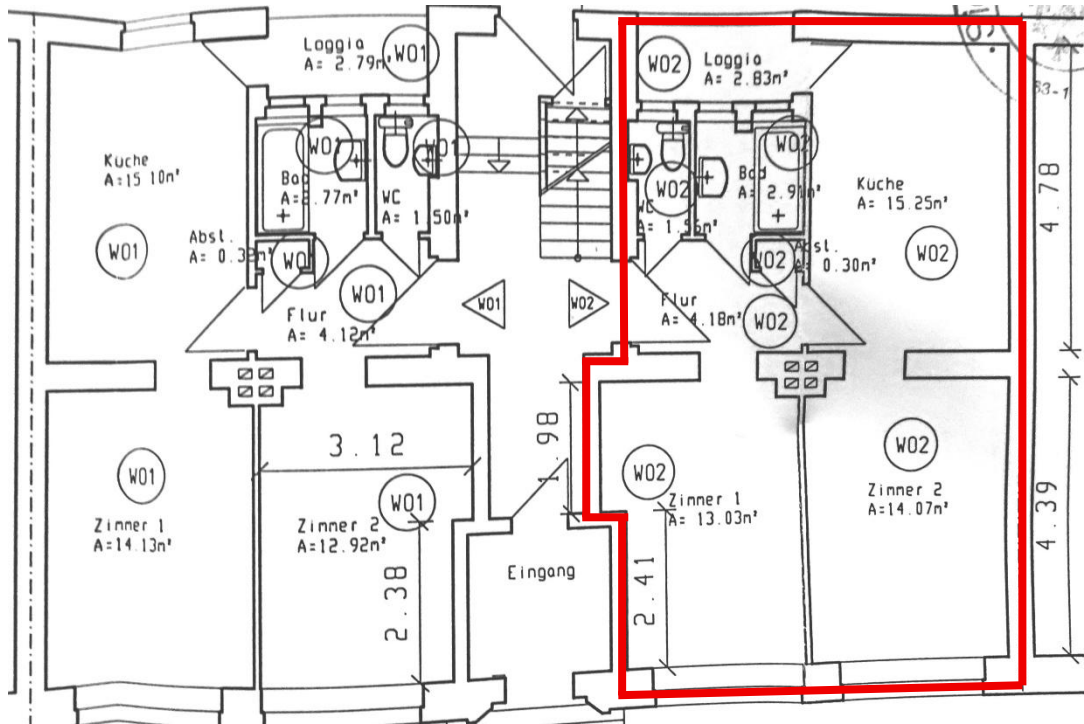
Grundrisskizze Wohnung ATP-Nr. 2 – Erdgeschoss rechts
