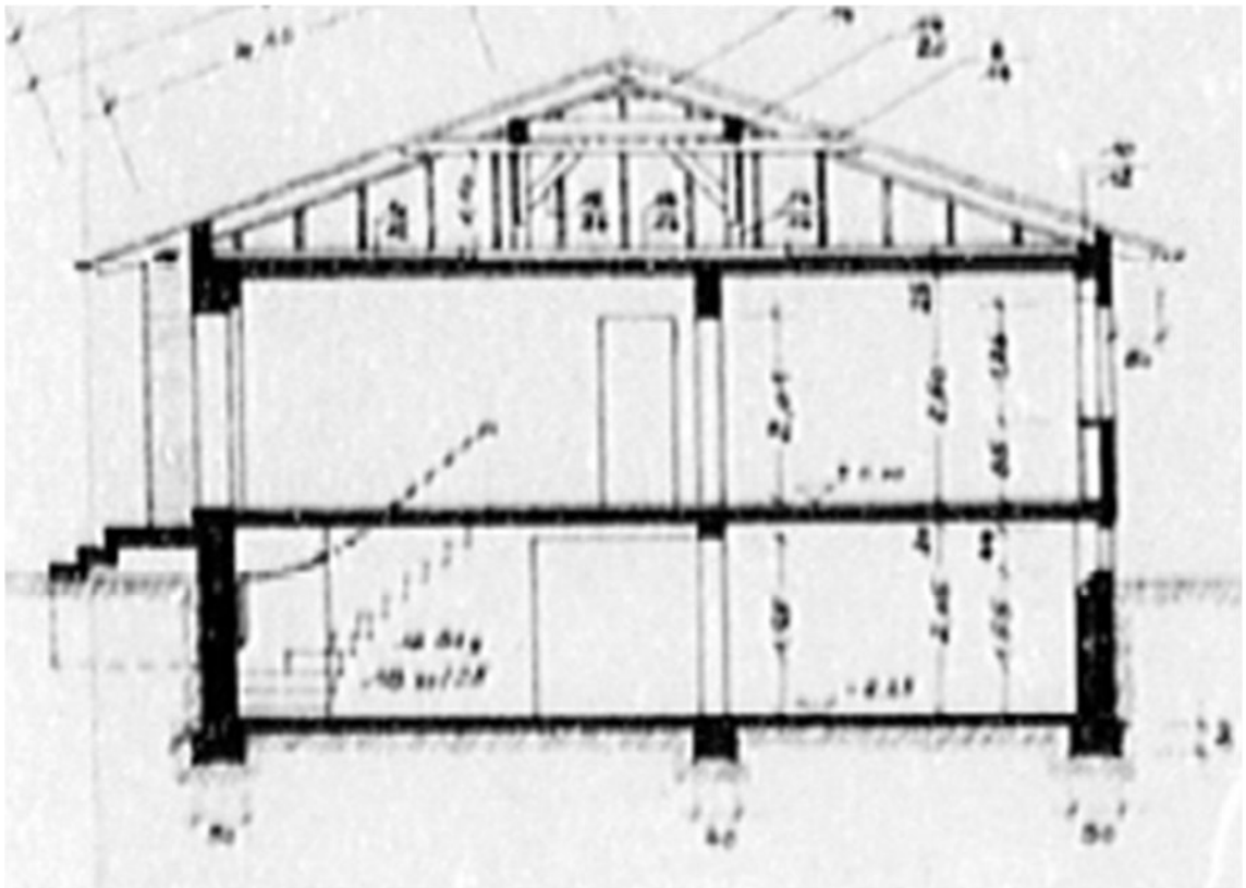
Querschnitt - Wohnhaus
