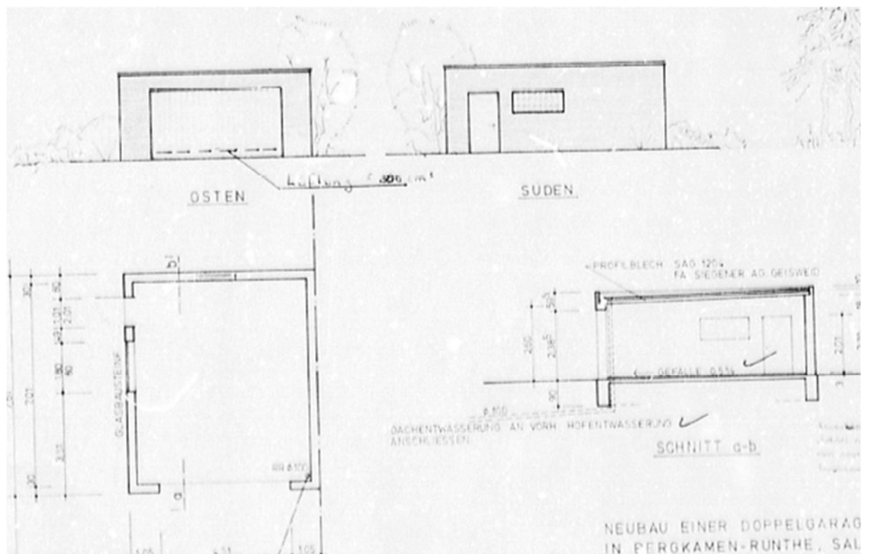
Doppelgarage
