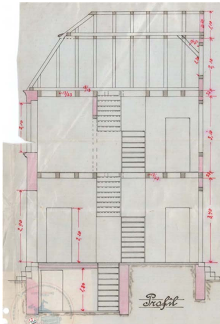
Schnitt
