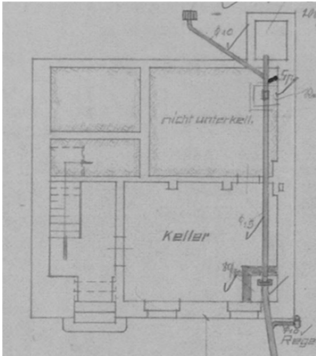
Kellergeschoss
